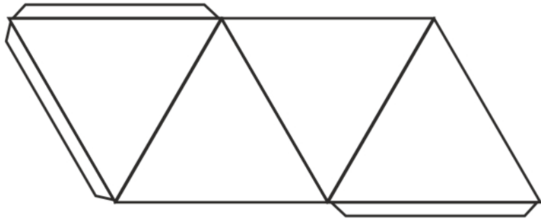
Şekil 12.24. Bireysel etkinlik için Tetrahedron ambalaj açılımı.
